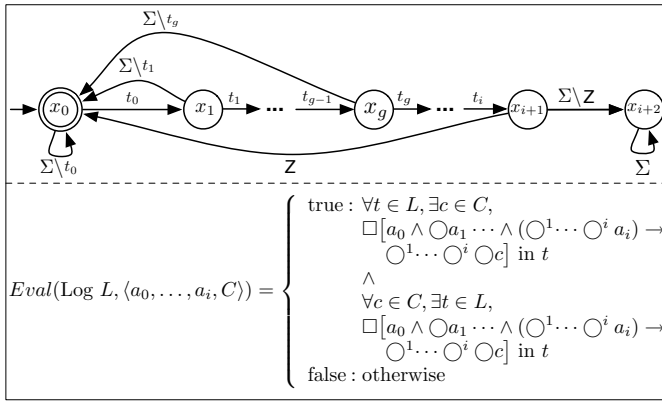
Fig. 10. The k\text{Tails}(k=i) property type.
